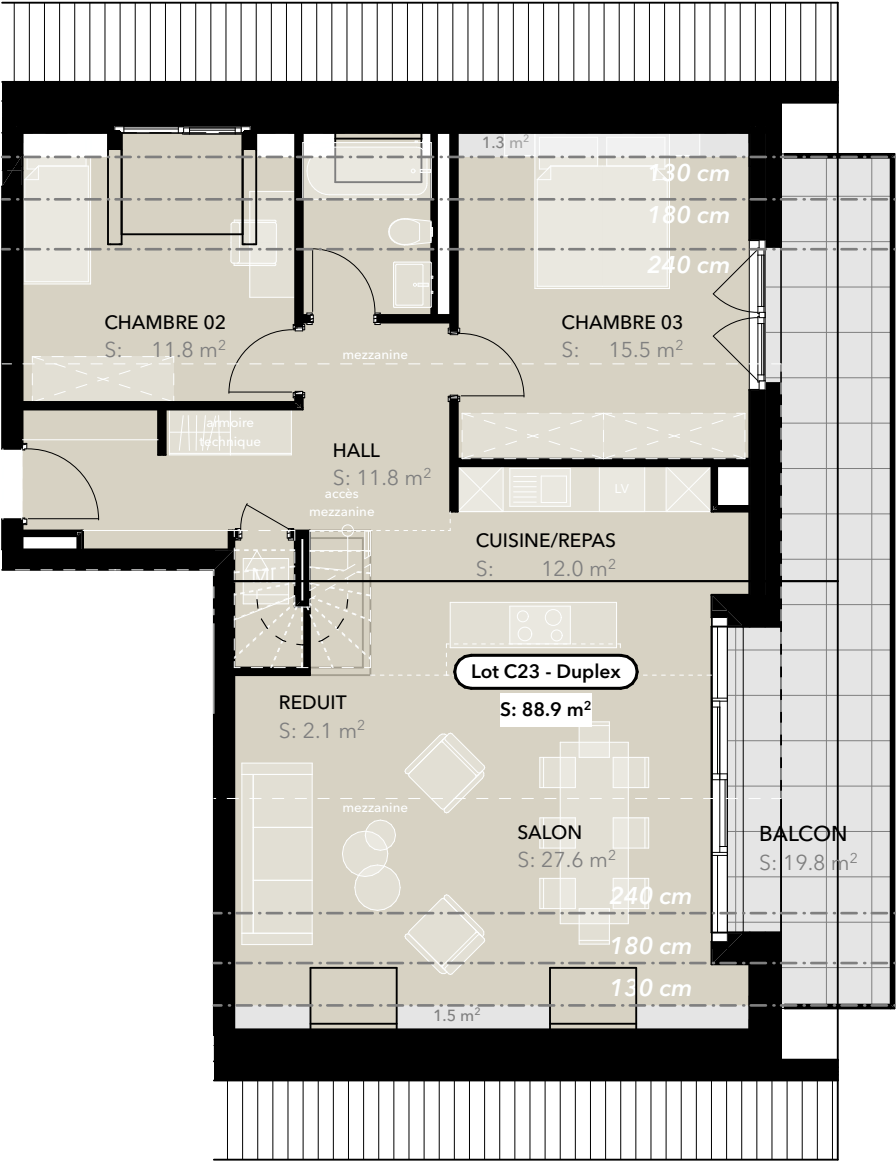
Combles - C23
